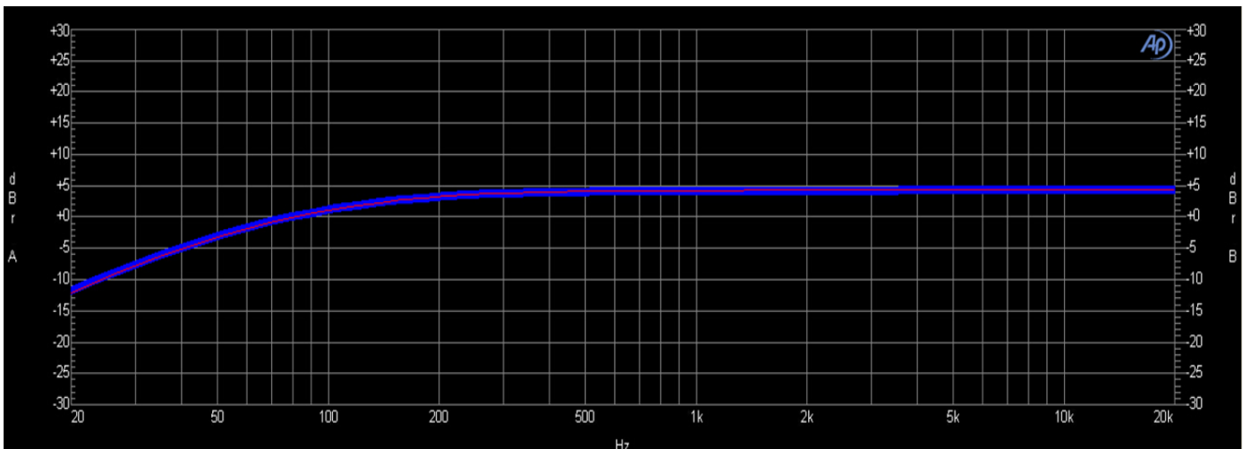
Av VS. Frequency @ R_L=32\Omega
