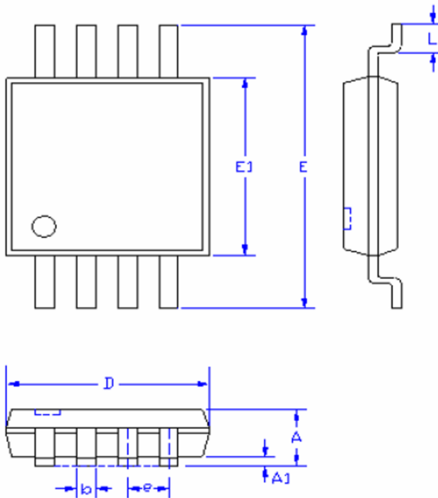
MSOP8
